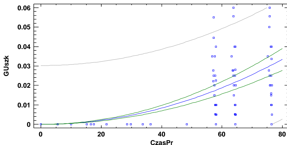
Rys. 4. Wykres zmian gęstości uszkodzeń dla różnych odcinków taśm na przenośniku o długości 2km z dobraną funkcją kwadratową Y = b \cdot X^2 ( b=0.00000521741 , R^2=67.3\% ).
