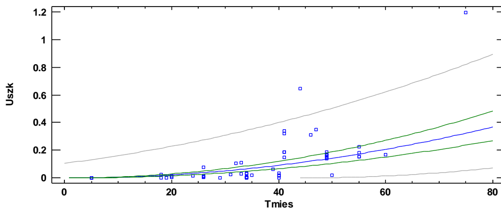
Rys. 2. Zmiany poziomu gęstości uszkodzeń z dobranym modelem funkcji kwadratowej (2).
