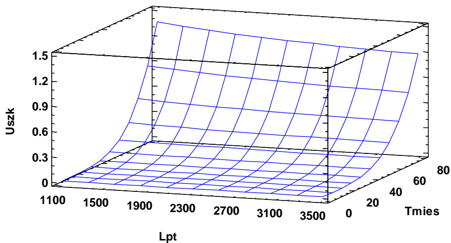
Rys. 7. Wykres powierzchni odpowiedzi dla regresji nieliniowej gęstości uszkodzeń od długości pętli taśm i dotychczasowego czasu pracy odcinków taśm podanego w miesiącach.
