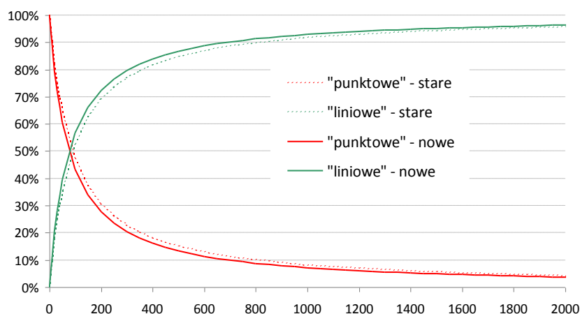
Rys. 5. Procentowy udział „punktowych” i liniowych” czynników uszkodzających w procesie zużywania się taśmy w zależności od długości przenośnika.
