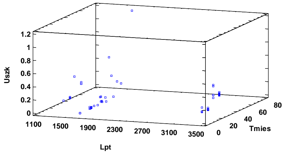
Rys. 6. Wykres punktowy gęstości uszkodzeń (Uszk) w zależności od długości pętli taśm (Lpt) i dotychczasowego czasu pracy odcinków taśm podanego w miesiącach (Tmies).
