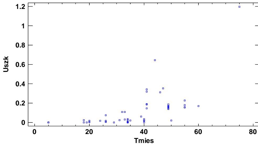
Rys.1 Zmiany gęstości uszkodzeń odcinków taśm w zależności od czasu ich pracy (w mies.).
